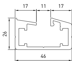
Profilo binario inferiore ribassato
